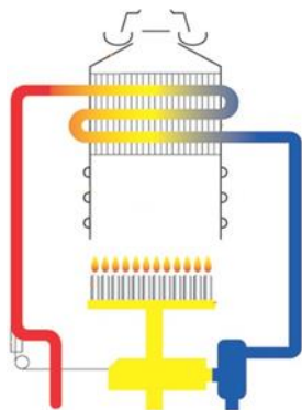
DIAGRAMA FUNCIONAL
